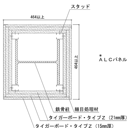
独立柱の水平断面図
