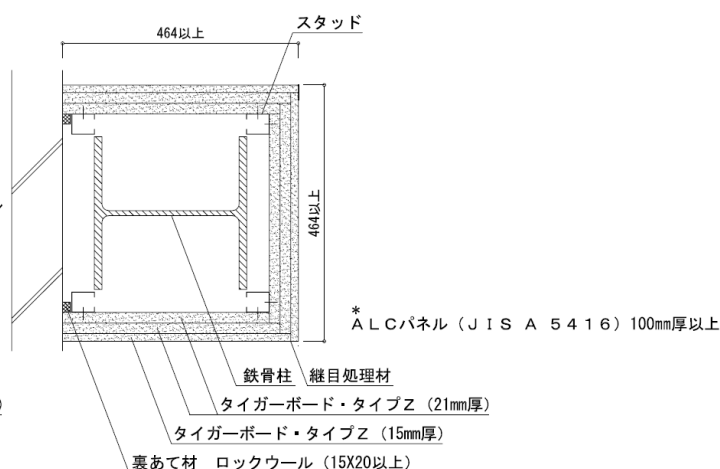
合成柱の水平断面図
